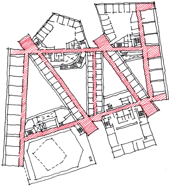
图3: 天津茱莉亚学院二层平面图
